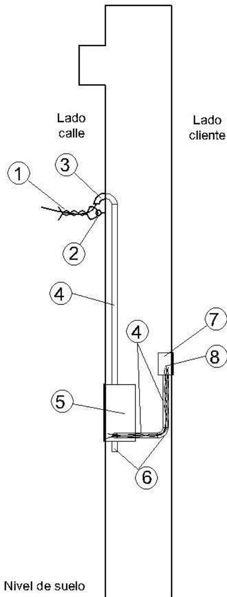
Vista lateral
