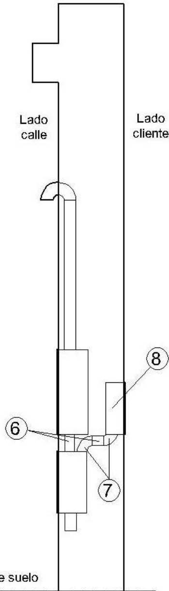
Vista lateral
